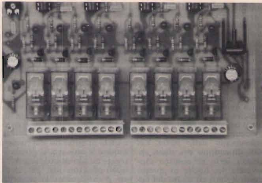
Particolare relé.
