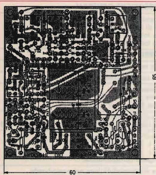
figura 5 Basetta RF.
