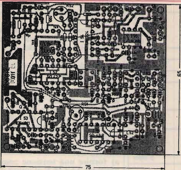
figura 4 Basetta AF/IF.
