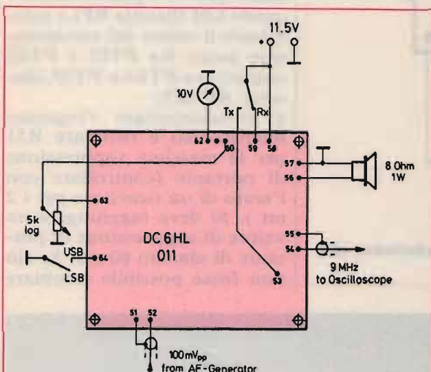
figura 7 Come collaudare il modulo AF/IF.
